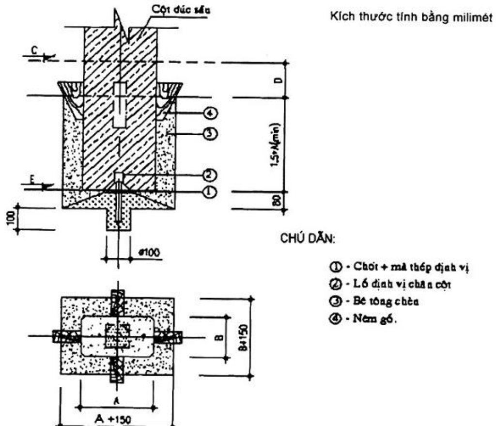
Hình 4 - Ví dụ lắp cột vào móng cốc
