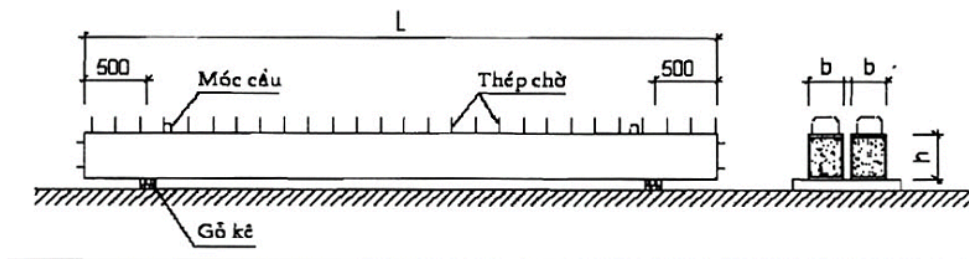
Hình 2 - Kê xếp dầm bê tông cốt thép ứng lực trước
